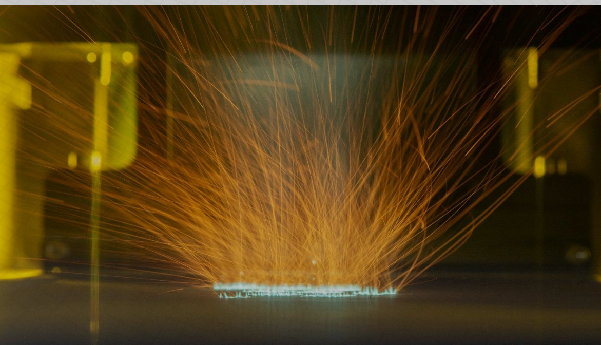
Drukarka 3D do druku metalu, PROCES DRUKU
