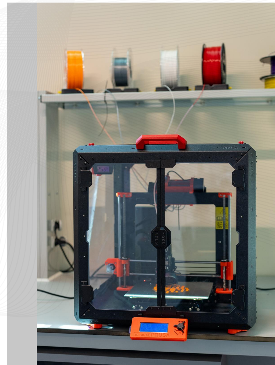
Drukarka 3D do druku z polimerów
